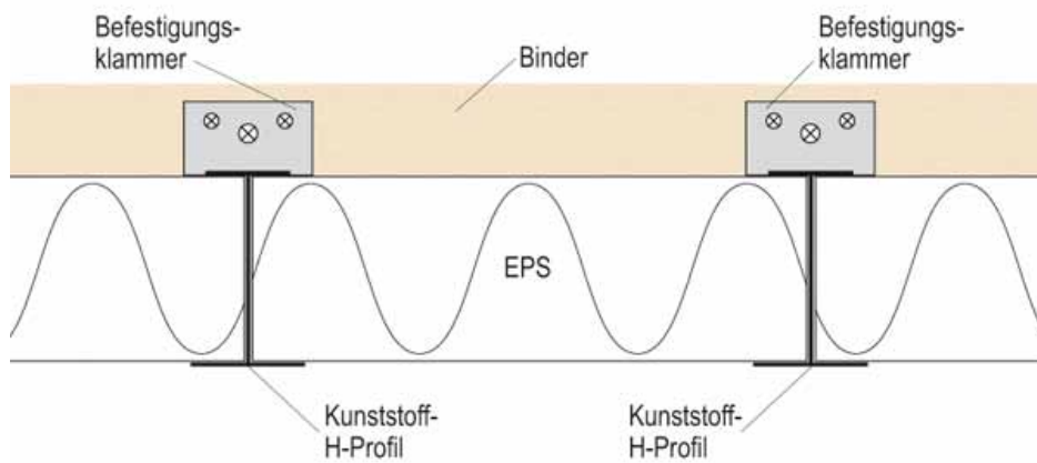
Variante mit H-Profil – mit abgewinkelten Befestigungsklammern
