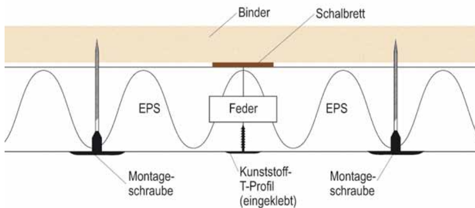
Variante mit Nut und Feder – kältebrückenfrei – mit rückseitigem Schalbrett zur Abdichtung der Fuge
