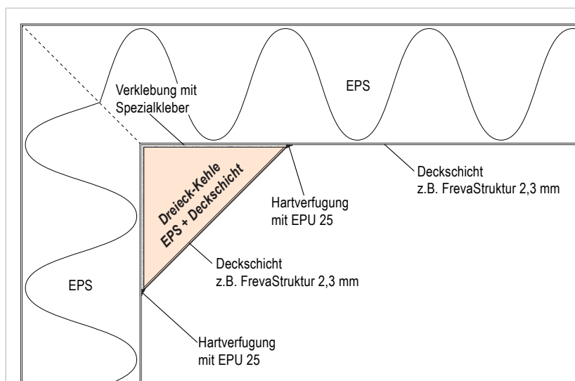
Dreieck-Kehle 2-teilig für Anschluss Decke/Decke/Wand
